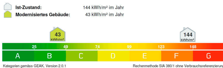
Heizenergiebedarf vor und nach Sanierung
